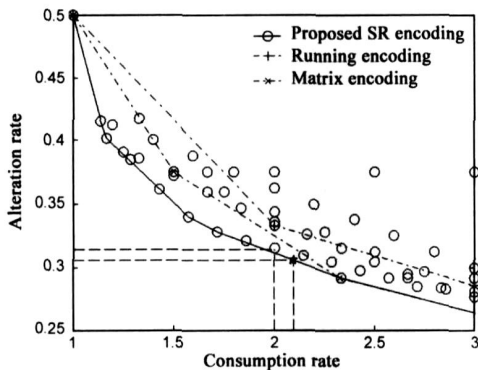
图 1 占用率在 [1, 3] 之间 k \leq 7 的密写编码性能. 实线代表组合编码可获得的最佳性能. 当占用率为 2.110 时, 组合方法获得的最小更改率为 0.305, 优于非组合方法的最小更改率 0.315. 两条虚线分别代表矩阵编码和游动编码的性能, 劣于本文方法性能
